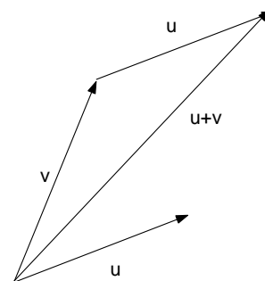
KUVA 1. Vektorisumma u + v
